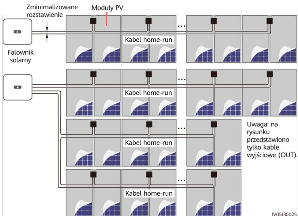
Rysunek 2-4 Wymagane prowadzenie kabli
