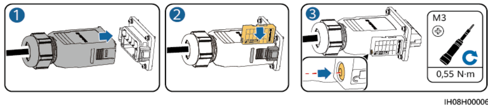
Rysunek 5-9 Podłączanie złącza AC
