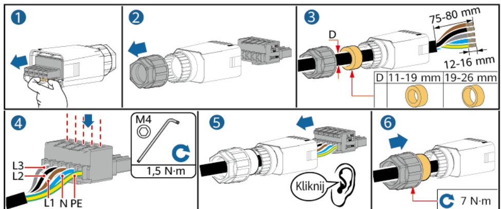
Rysunek 5-8 Kabel pięciożytowy (L1, L2, L3, N i PE)
