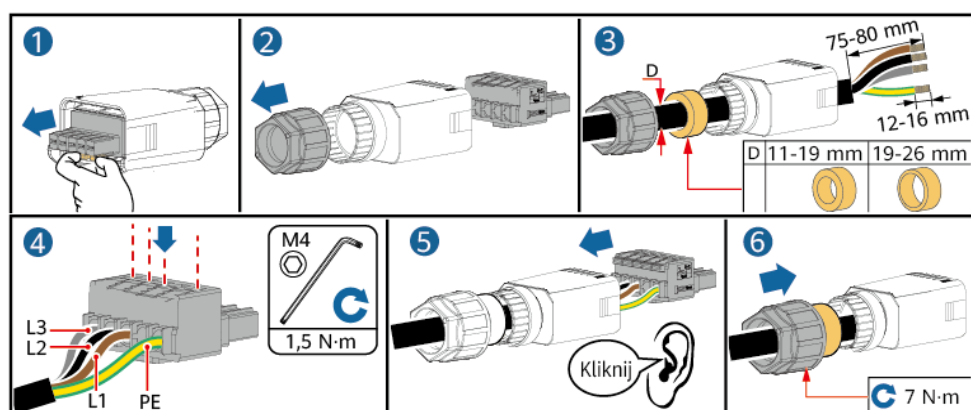
Rysunek 5-6 Kabel czteryżyłowy (L1, L2, L3 i PE)
