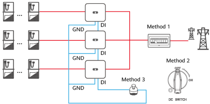
Rysunek E-1 Metody wyzwalania szybkiego wyłączenia
