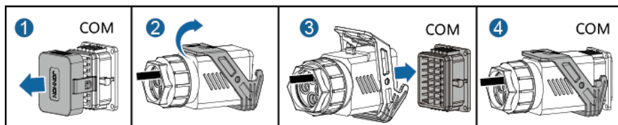
Rysunek 5-38 Zabezpieczenie złącza kabla sygnałowego
