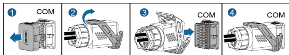
Rysunek 5-36 Zabezpieczenie złącza kabla sygnałowego
