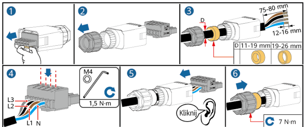
Rysunek 5-7 Kabel czteryżytowy (L1, L2, L3 i N)
