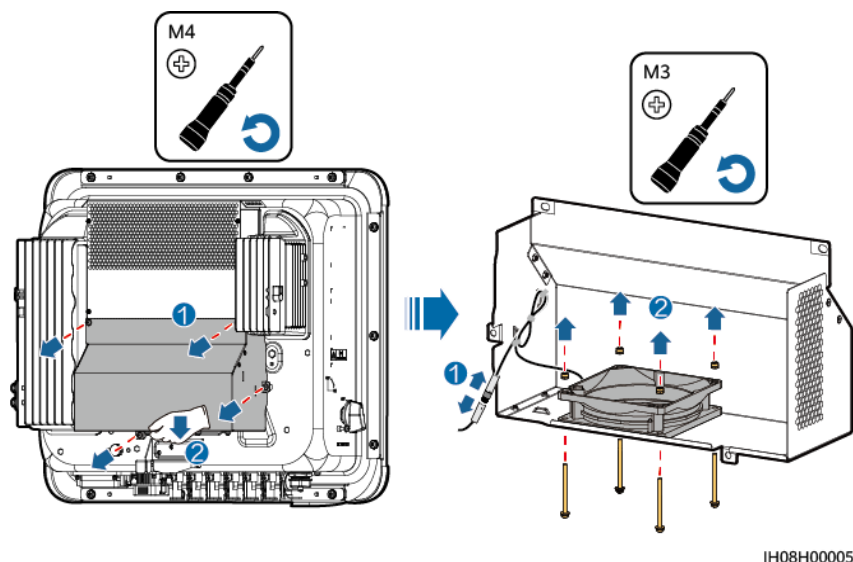
Rysunek 8-1 Wymywanie wadliwego wentylatora
