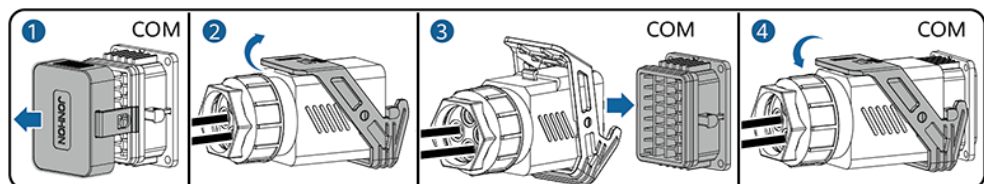
Rysunek 5-21 Zabezpieczanie złącza kabla sygnałowego
