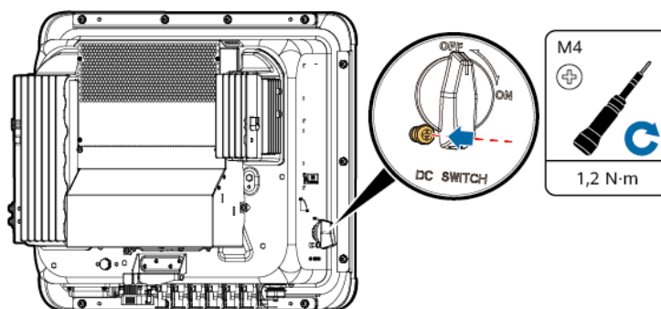
Rysunek 4-11 Instalacja śruby zabezpieczającej przełącznika DC
