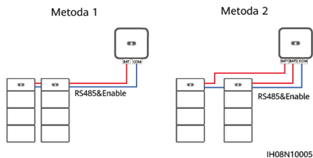
Rysunek 2-5 Podłączanie falownika do dwóch baterii
