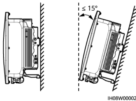
Rysunek 4-5 Kąt montażu
