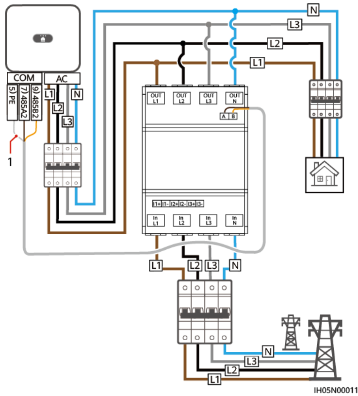
Rysunek 5-26 Bezpośrednie połączenie trójfazowe, czterożyłowe (połączenie sieciowe Smart Dongle)
