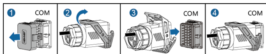
Rysunek 5-32 Zabezpieczenie złącza kabla sygnałowego
