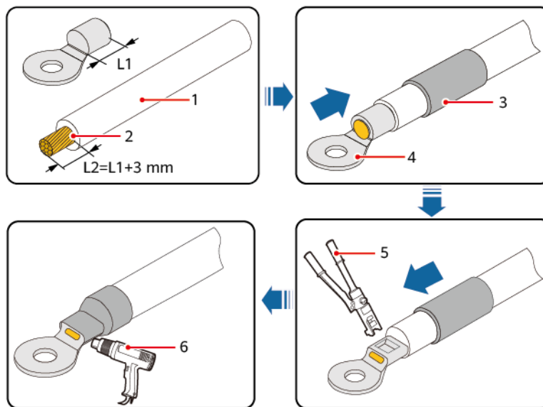
Rysunek 5-2 Zaciśnięcie zacisku OT
