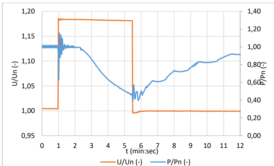
Obr.10.3: Křivka ORVT 1,18 U_n po dobu 4,5 s
