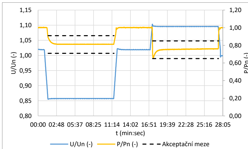
Obr.8.1: Napěťová stabilita
