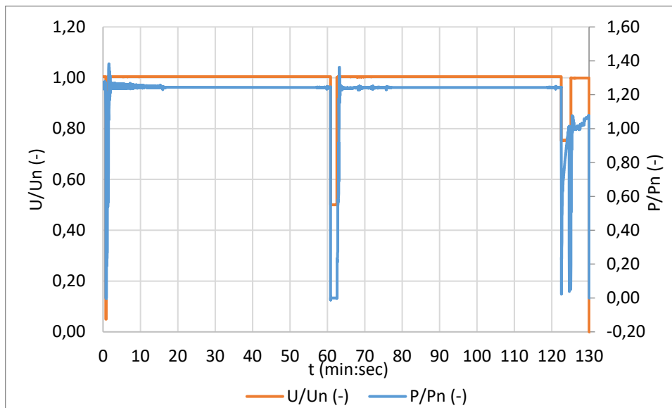
Obr.9.2: Křivka URVT – naměřeno
