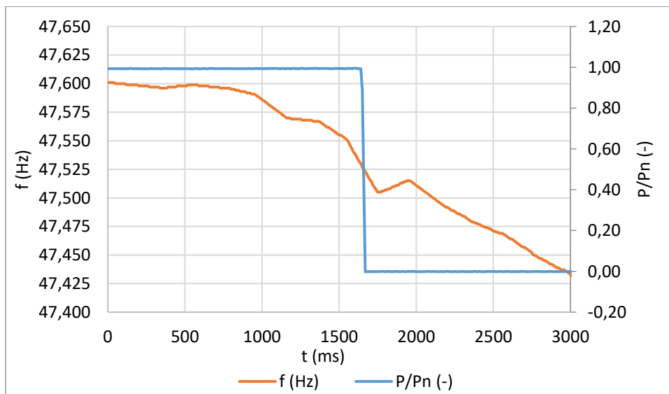
Obr.12.10: Podfrekvenční ochrana
