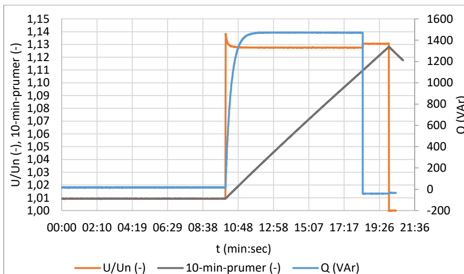
Obr.12.4: 10 min ochrana
