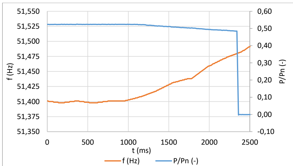
Obr.12.9: Nadfrekvenční ochrana
