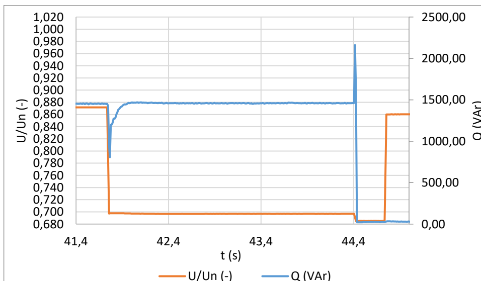
Obr.12.6: Podpětová ochrana 1. stupeň – detail
