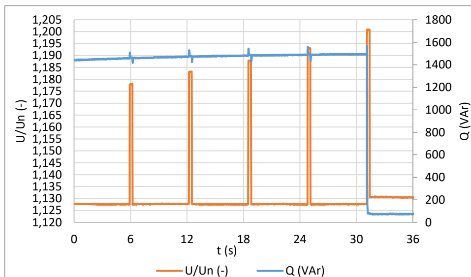
Obr.12.1: 3. stupeň nadpětí ochrany – impulzní rampa
