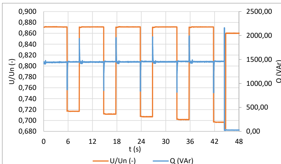
Obr.12.5: Podpětová ochrana 1.stupeň
