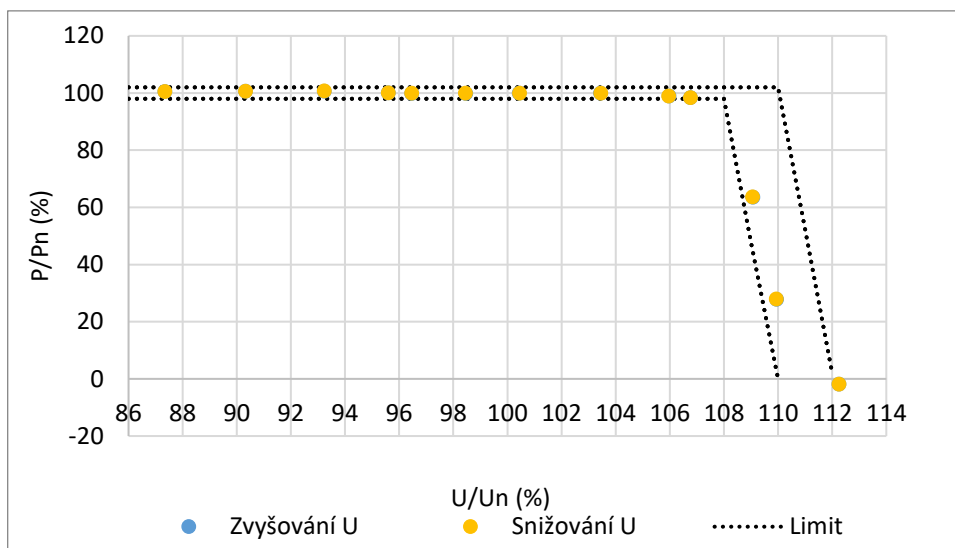
Obr.11.2: P(U) – vyhodnocení
