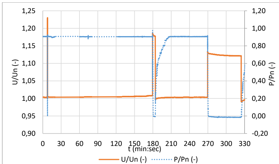
Obr.10.2: Křivka ORVT
