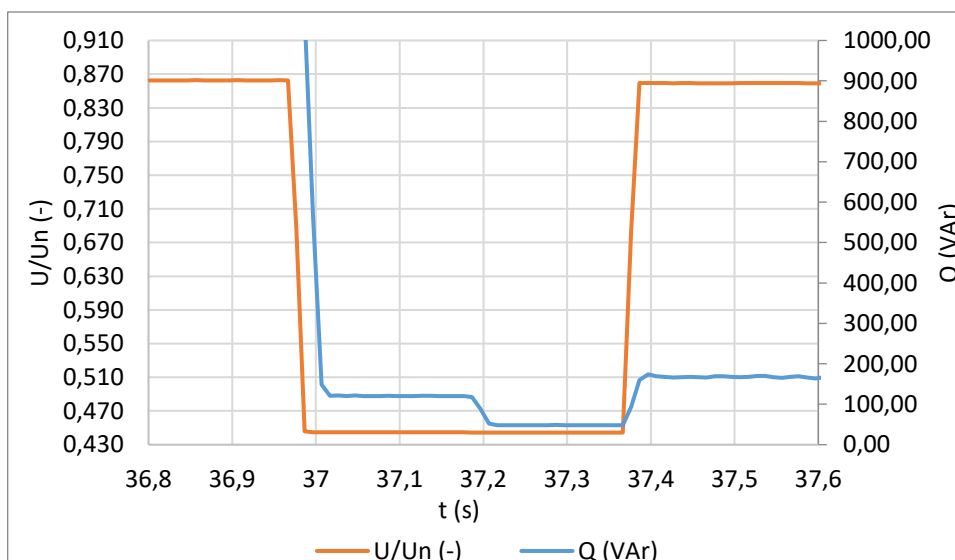
Obr.12.8: Podpětová ochrana 2.stupeň – detail
