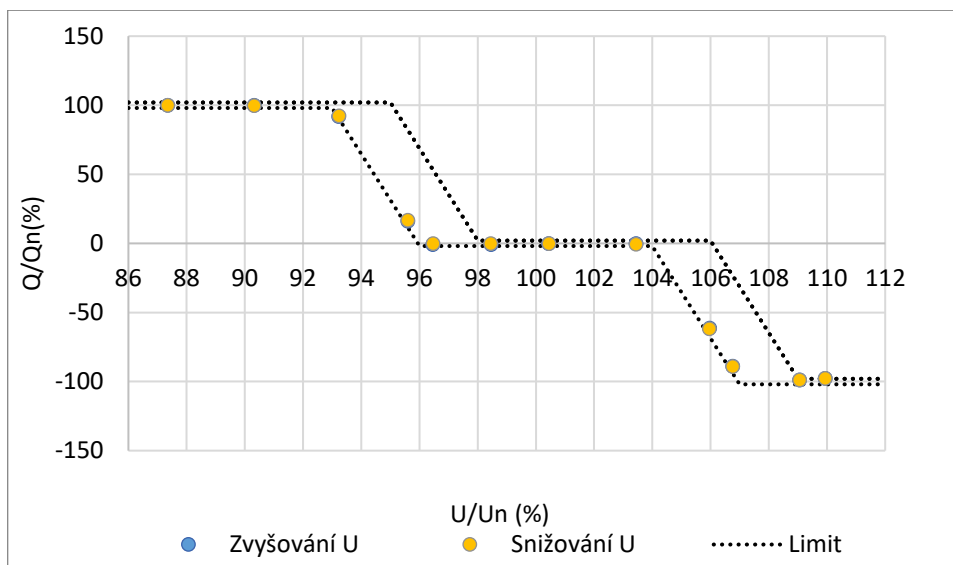
Obr.11.4: Q(U) – vyhodnocení
