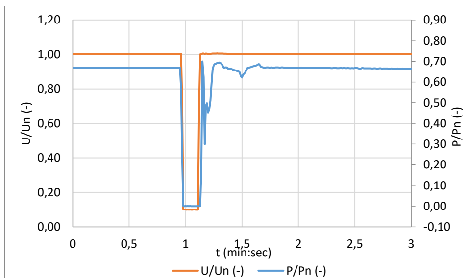
Obr.13.1: Obnovení činného výkonu po krátkodobém poklesu napětí
