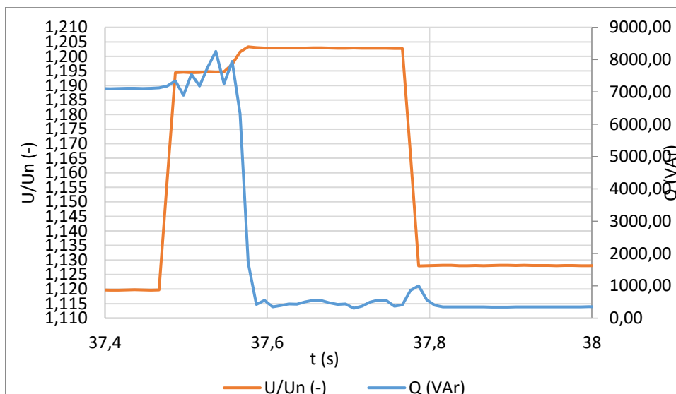
Obr.12.2: 3. stupeň nadpětové ochrany – detail
