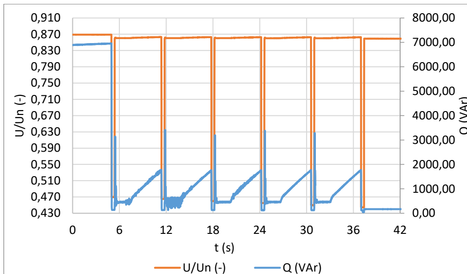
Obr.12.7: Podpětová ochrana 2.stupeň
