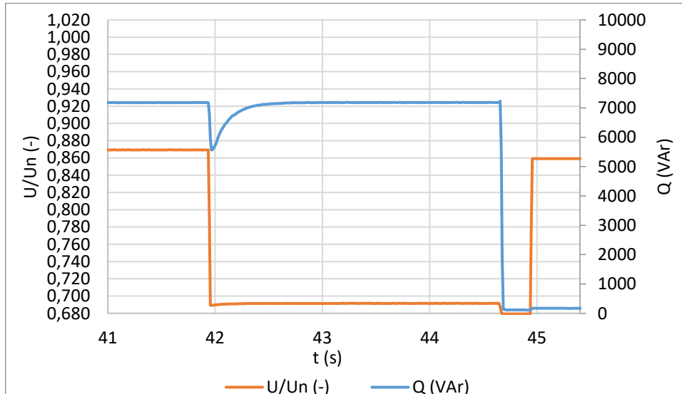
Obr.12.6: Podpětová ochrana 1. stupeň – detail
