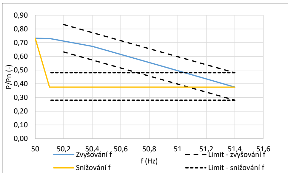
Obr.3.2: P(f) křivka při nadfrekvenci – 73 % výkonu
