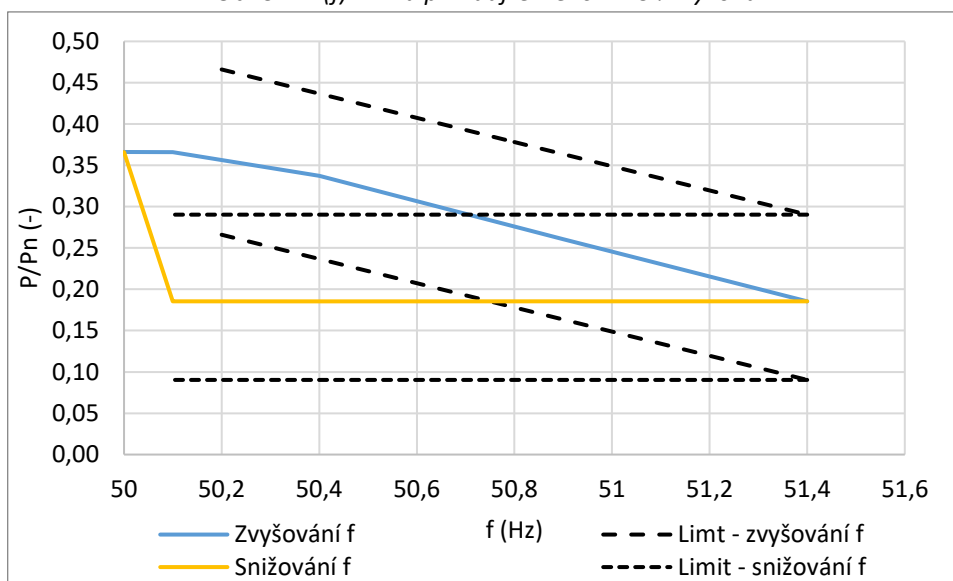
Obr.3.3: P(f) křivka při nadfrekvenci – 37 % výkonu
